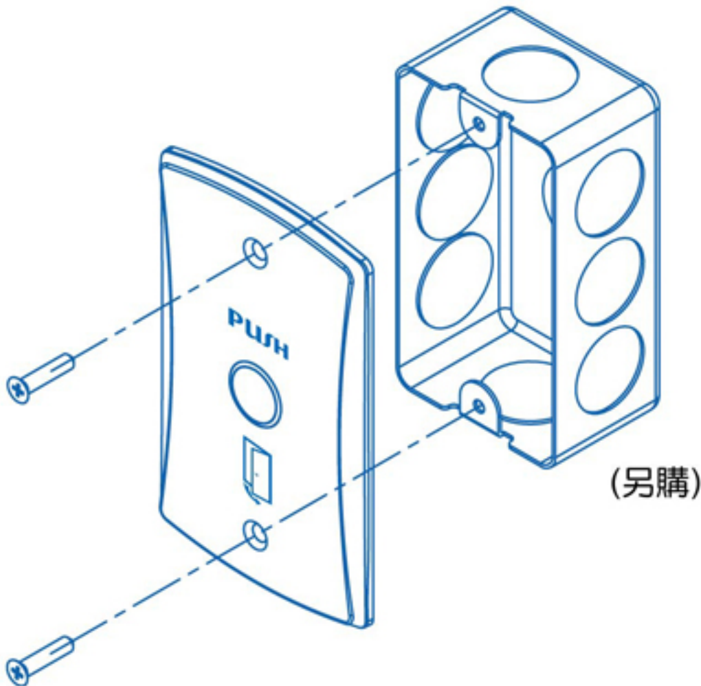
型號:PBT-09/IRA 尺寸:115(L) x 70(W) x 5(H)mm (通電時: 紅燈 / 感應時: 藍燈) 可暫態/常態切換 接點:N.O. / N.C. / COM.
